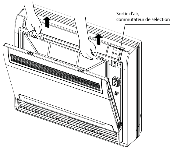
Fig. 7 – L'air est soufflé depuis les sorties supérieure et inférieure Retirez le filtre à air
